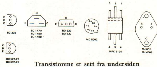
Transistorene er sett fra undersiden
