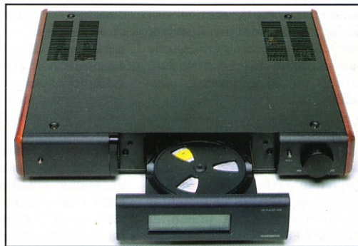
PLATEILEGGET på Tandberg CD-spilleren. Skuffen med hele drivverket og laser kommer ut. For å stabilisere platen legger man på en clamp.
