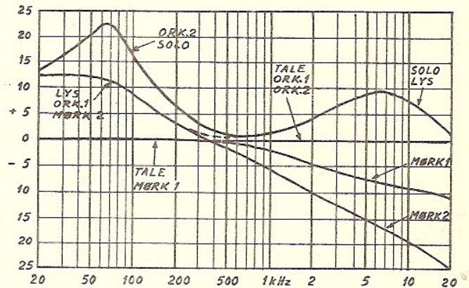
Fig. 6. Frekvenskurver for LF del målt i stilling Bånd og Gram. Signalspenning 0.25 volt. Volumkontroll -30 dB (stilling ca. 3\frac{1}{2} ). Kurvene gjelder også i stilling FM når senderen har standard preemphasis. (50 \mu s).
