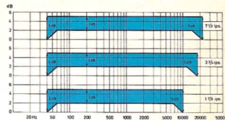
De färgade fälten visar toleransområden för frekvensgång mätt efter DIN 45511.
