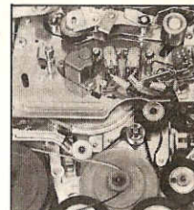
Tachometerhjulet kontrollerar att motorhastigheten alltid är korrekt.
