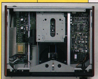
CD-spiller
