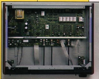
Effektforsterker.
